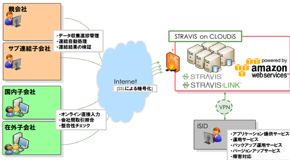
<STRAVIS on CLOUDiS システム構成図>
